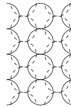
fcc (110)
