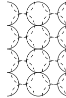
fcc (110)
